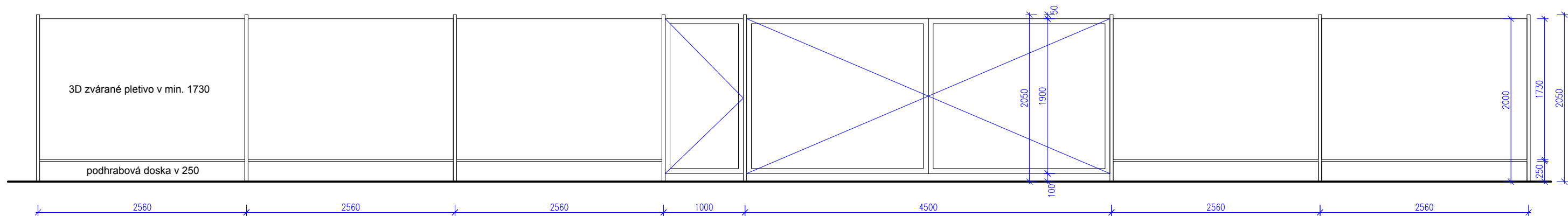
POHLAD NA OPLOTENIE S BRÁNOU A3 + B5 - POHLAD SEVERNÝ
